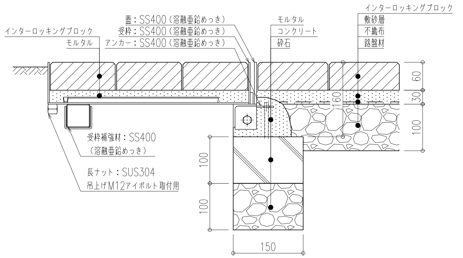
施工参考拡大図
